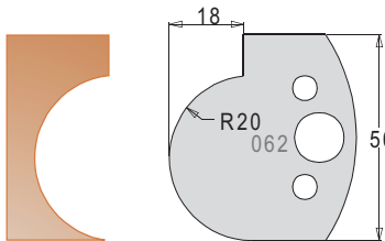
Knife 3306250 Limiter 3406250
