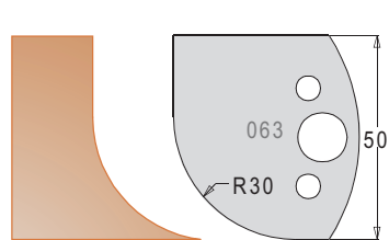
Knife 3306350 Limiter 3406350
