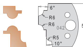
Knife 3304250 Limiter 3404250
