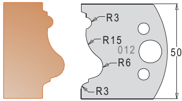
Knife 3301250 Limiter 3401250
