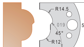
Knife 3301950 Limiter 3401950
