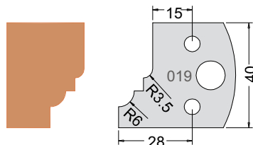
Knife 3301940 Limiter 3401940
