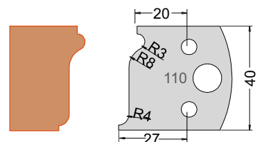
Knife 3311040 Limiter 3411040
