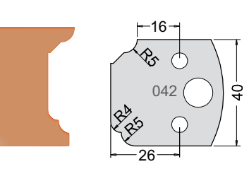
Knife 3304240 Limiter 3404240
