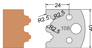
Knife 3310840 Limiter 3410840
