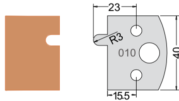
Knife 3301040 Limiter 3401040
