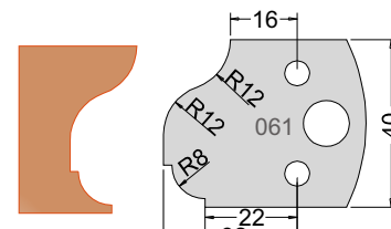
Knife 3306140 Limiter 3406140
