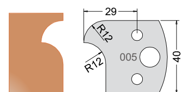
Knife 3300540 Limiter 3400540
