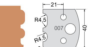
Knife 3300740 Limiter 3400740
