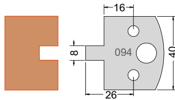
Knife 3309440 Limiter 3409440
