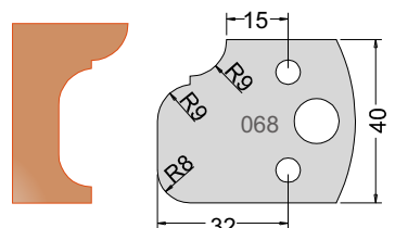
Knife 3306840 Limiter 3406840
