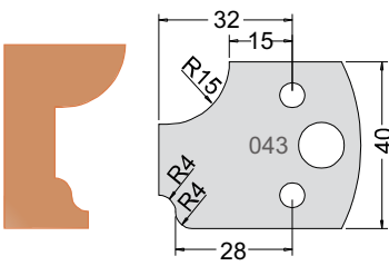
Knife 3304340 Limiter 3404340
