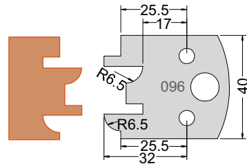
Knife 3309640 Limiter 3409640
