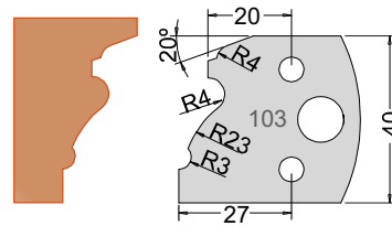
Knife 3310340 Limiter 3410340
